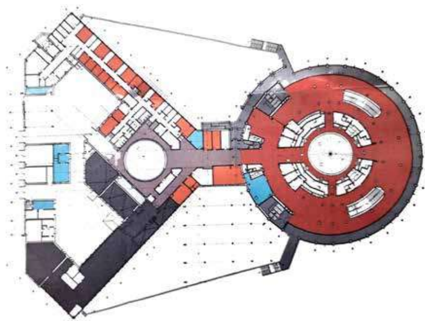
Figura 3. Circul de Stat. Plan ansamblu. Cota ± 0.00 (Arhiva B.A.C.U.)
