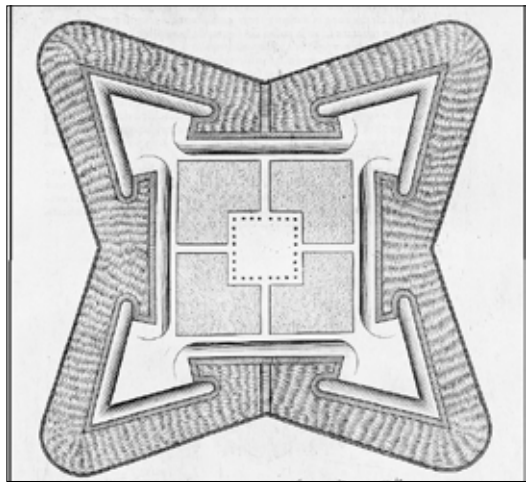
Fig. 5. Planul careului bastionar (după Jean Errard de Bar-Le-Duc)
