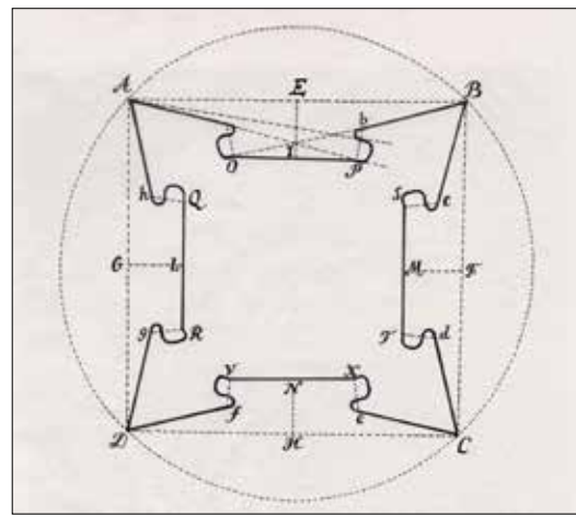
Fig. 4. Planul fortului pătrat cu patru bastioane de colț (desenul autorului după Vauban și V.I. Suvorov)
