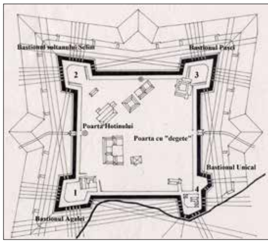
Fig. 3. Planul cetății bastionare a Chilie, probabil după 1797 (desenul autorului după un relevu din AMIRM atribuit lui F. Kauffer)
