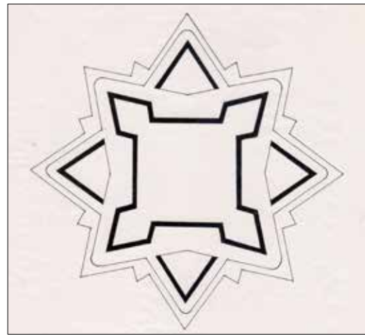
Fig. 6. Planul careului bastionar (desenul autorului după Louis de Cormontaigne)
