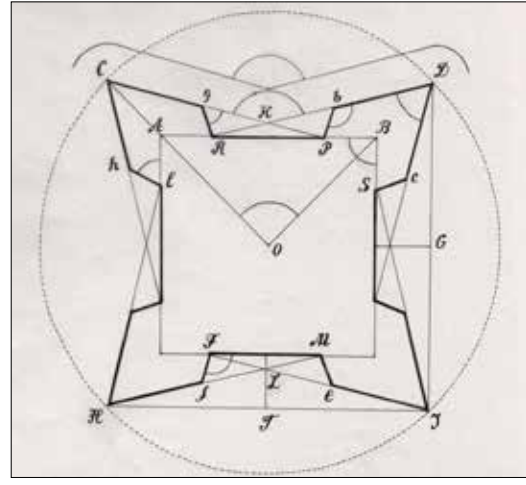
Fig. 8. Planul fortului rectangular bastionar cu indicarea unghiurilor (desenul autorului după Vauban)
